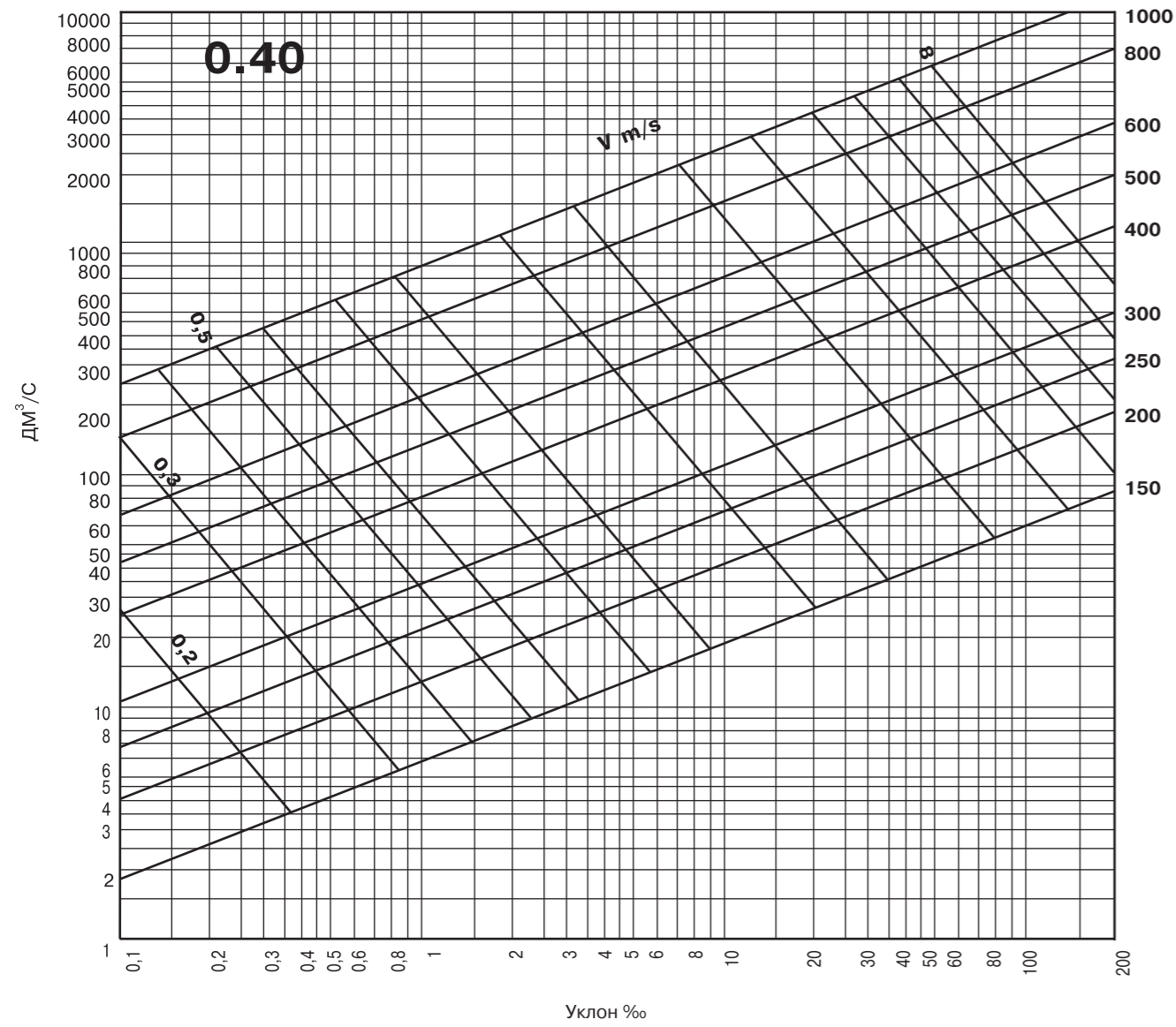
Рисунок Б.1 - Номограмма для определения гидравлического расчета самотечных канализационных трубопроводов
